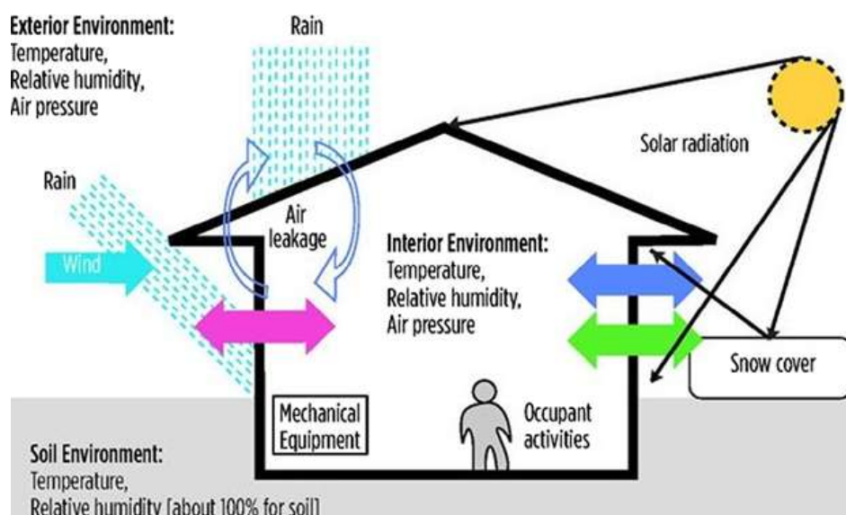
شکل ۲. متغیرهای وابسته به محیط و ساختمان که بر شرایط داخلی ساختمان‌ها تأثیر گذارند
