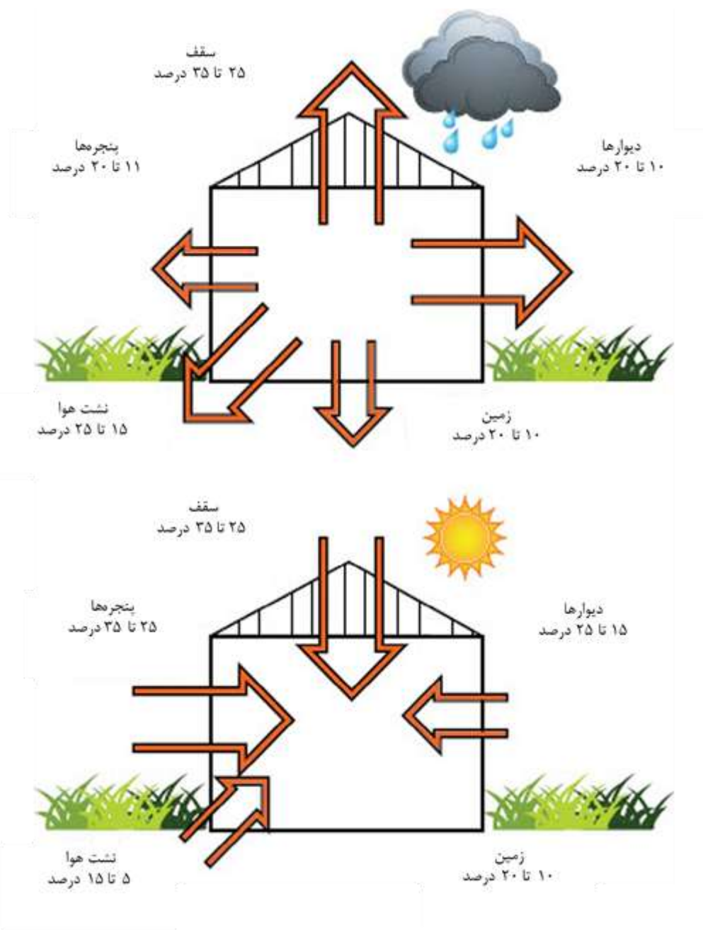
شکل ۱. جریان حرارتی در یک خانه‌ی بدون عایق بندی واقع در منطقه آب و هوایی خنک
