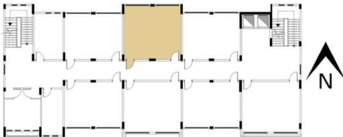
شکل ۵. پلان استاندارد طبقه همکف نشان دهنده ی سالن مطالعه ی ساختمان برنامه ریزی فضایی، دانشکده ی مهندسی دانشکده ادبیات دانشگاه شیراز
