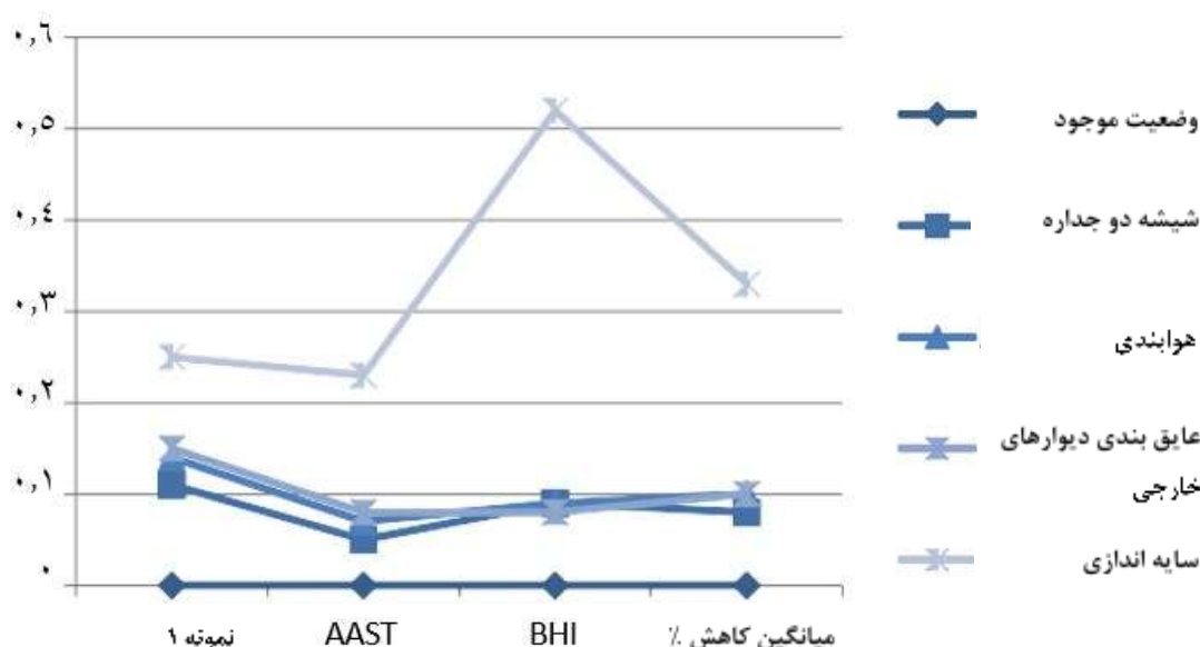
شکل ۱۱. مقدار انرژی کاهش یافته بر اساس هر یک از راهبردها
