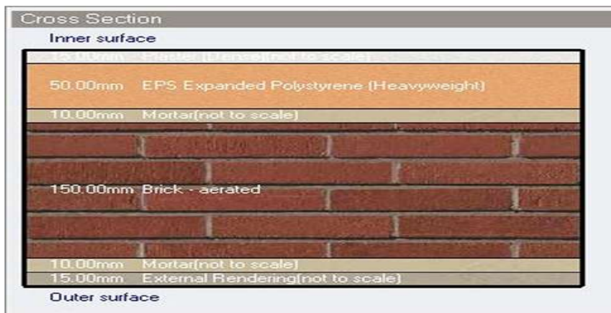
شکل ۹. مقطع لایه-های دیوار پس از اعمال متریال عایق بر دیوار موجود
